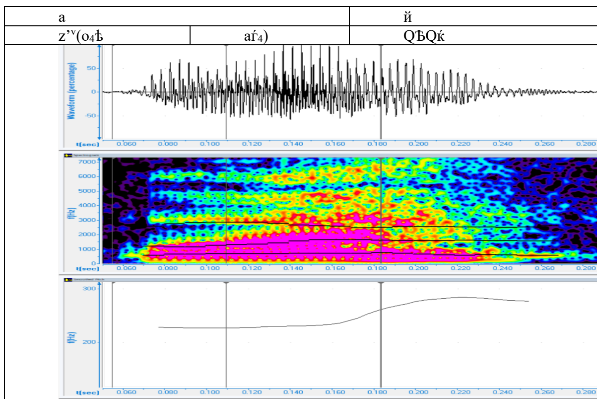
Рис. 2. Спектограмма и осциллограмма слова ай ‘луна’
