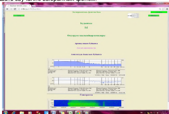
Рис. 1. Артикуляционные и экспериментальные характеристики фонемы [y].
