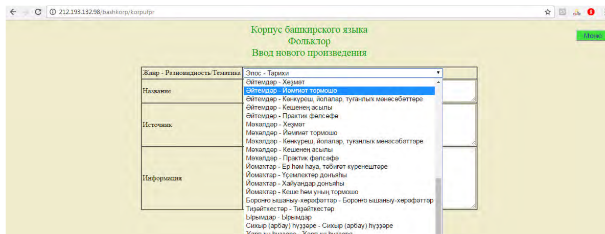
Рис. 2. Блок администратора, включающий программные средства для ввода текстов.
